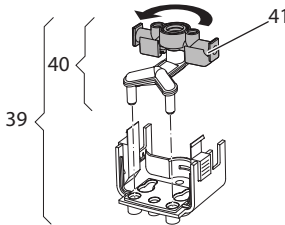
Afb. 21: Toevoer draaien
