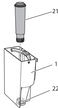
Joon. 15: Veefiltri paigaldamine/eemaldamine
