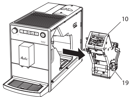
Fig. 12: Demontere bryggeenhet
