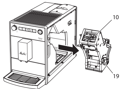
Bild 12: Demontera bryggenheten
