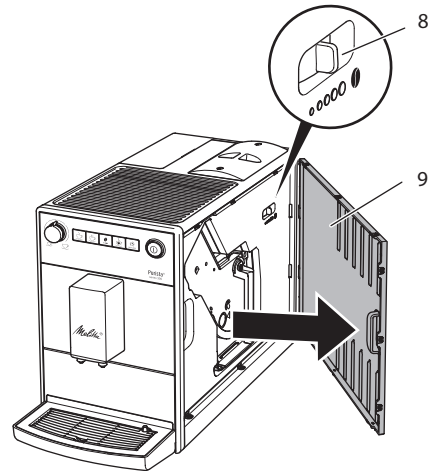
Рис. 11: Настройка тонкости помола
