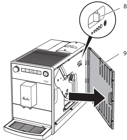
Fig. 11: Ajustar el grado de molienda
