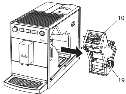
Fig. 12: Démontage de la chambre d'extraction
