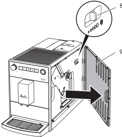
Fig. 11: Réglage de la finesse de mouture
