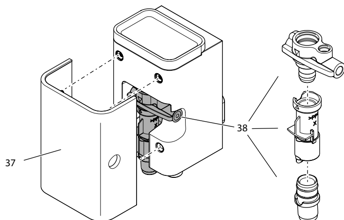
Fig. 19: Demontarea unității de lapte
