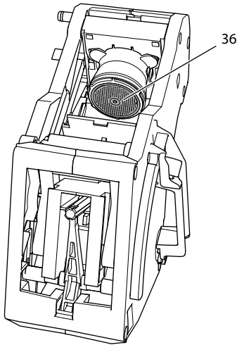
Abb. 18: Brühgruppe reinigen
