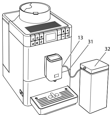
Fig. 11: Flaconul pentru lapte racordat
