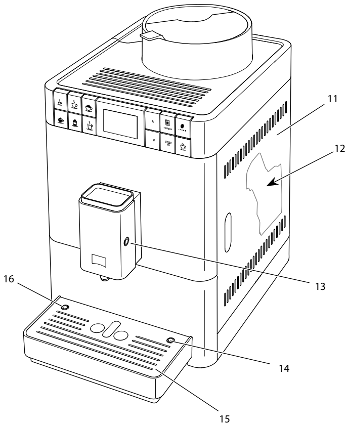
Fig. 2: Aparatul văzut din dreapta părții frontale
