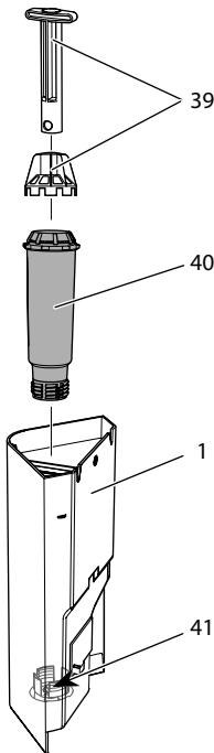
Fig. 20: Înșurubarea și deșurubarea filtrului de apă
