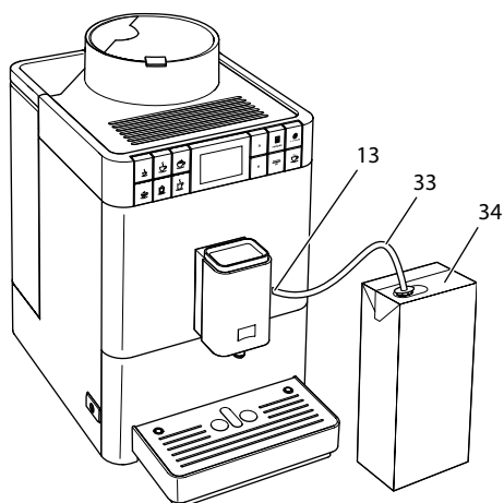
Att. 12: Pievienota veikalā pieejamā piena pakā
