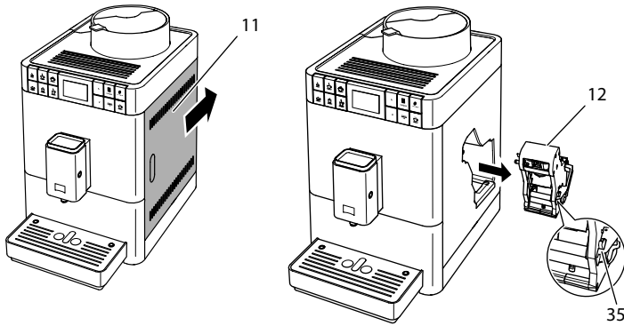
Fig. 17: Scoaterea unității de infuzare
