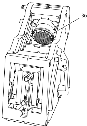
Fig. 18: Curățarea unității de infuzare
