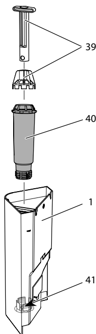
Fig. 20: Enroscar/denroscar el filtro de agua
