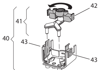
Kuva 19: Syöttöyksikön kääntäminen, 2
