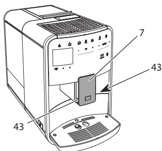
Abb. 23: Milcheinheit ausbauen, 1
