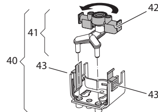
Joon. 19: Sissevooluava pööramine, 2
