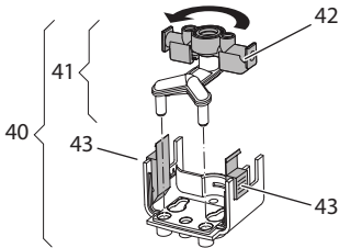
Bild 19: Vrida inloppet, 2
