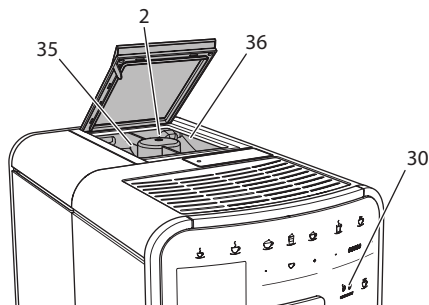
Att. 8: BARISTA TS divkameru kafijas pupiņu tvertne
