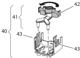
Fig. 19: Rotirea admisiei, 2
