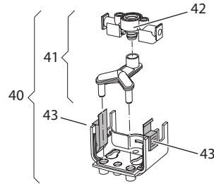
Şek. 24: Süt ünitesinin çıkarılması, 2
