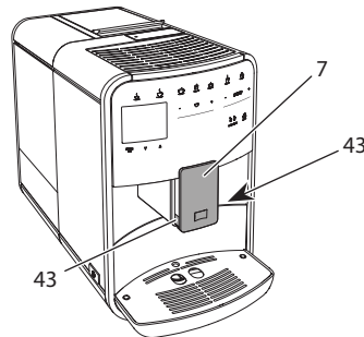
Afb. 23: Melkeenheid demonteren, 1
