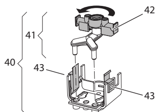
Fig. 19: Dreie innløp, 2
