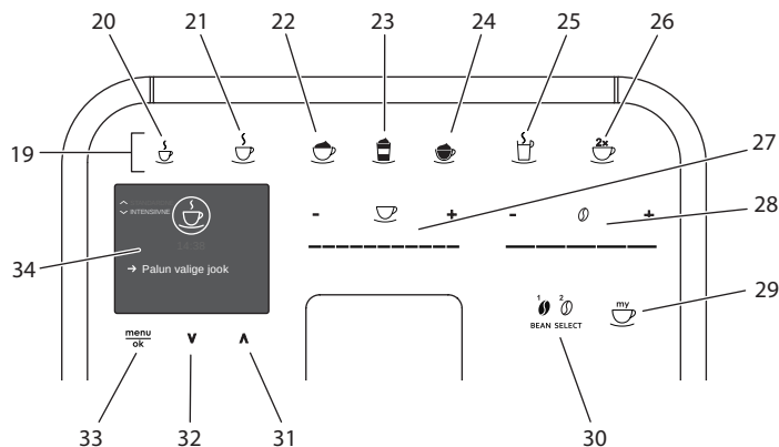
Joon. 3: Juhtpaneel
